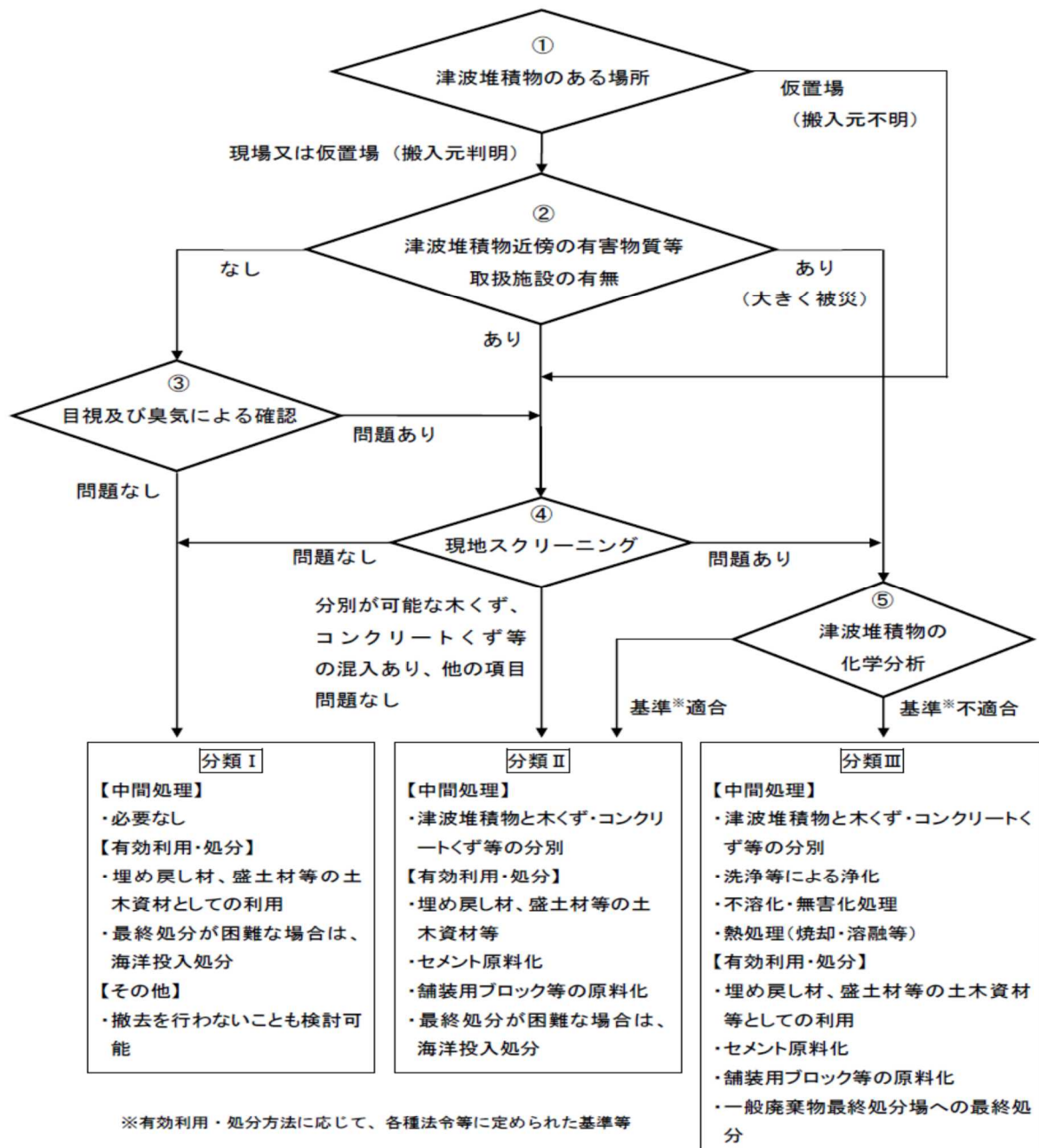
図 2-3-11-1 津波堆積物の基本的処理フローチャート
