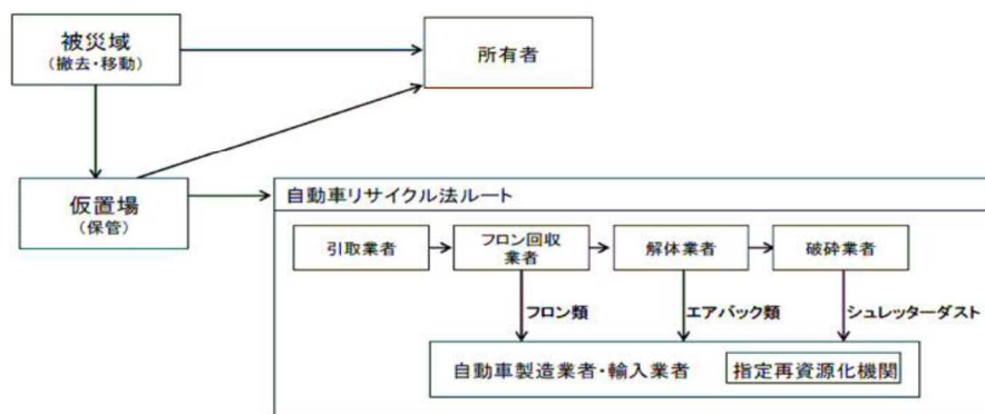
図 2-3-12-3 被災自動車の処理フロー
