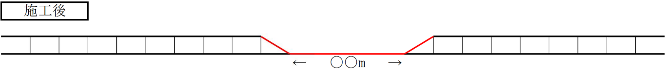
歩道舗装復旧断面図
