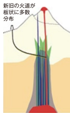
新旧の火道が板状に多数分布 火道掘削のイメージ図
